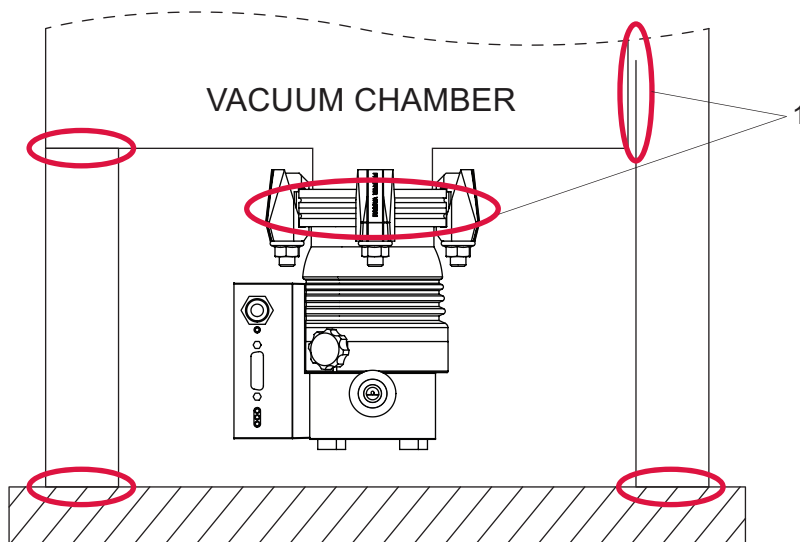
Abb. 4: Beispiel: Sicherheitsverbindungen
