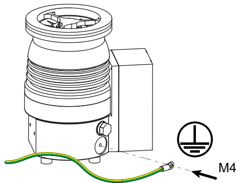
Abb. 17: Beispiel: Anschluss des Erdungskabels
