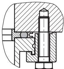
Abb. 8: Flanschverbindung ISO-K mit ISO-F, Pratze und Gewindebohrung
