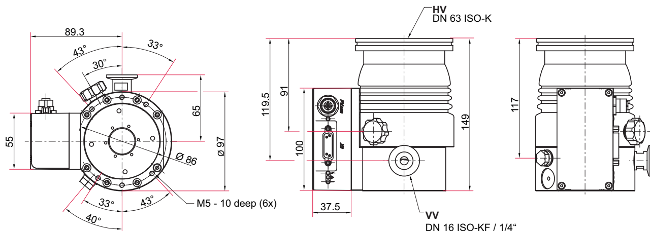
Abb. 23: Abmessungen HiPace 80 | DN 63 ISO-K
