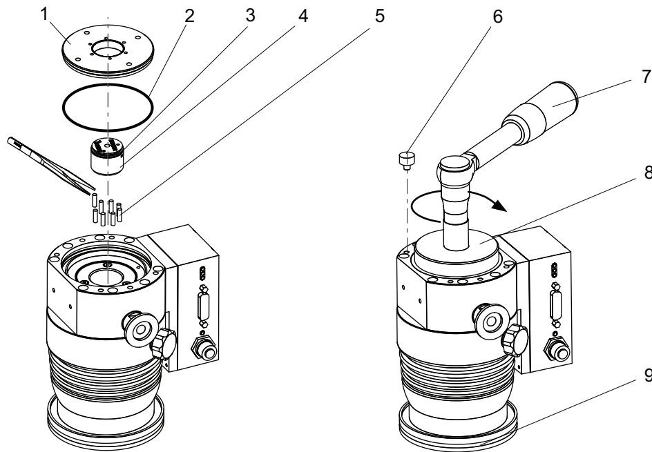
Abb. 20: Betriebsmittelspeicher montieren
