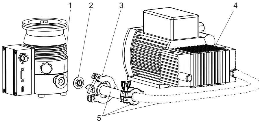
Abb. 15: Beispiel für den Vorvakuumanschluss an HiPace 80
