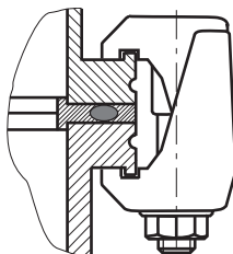
Abb. 7: Flanschverbindung ISO-K zu ISO-K, Klammerschraube
