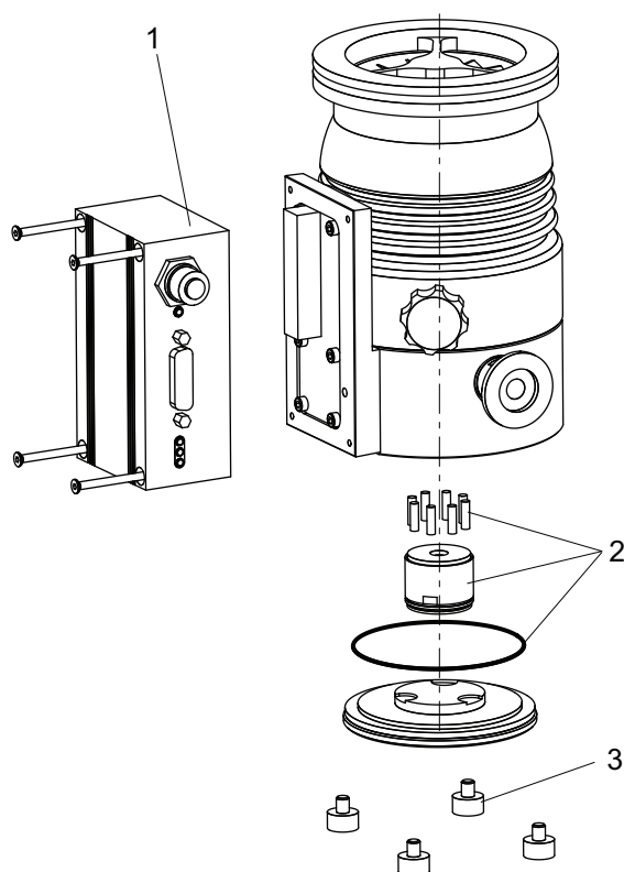
Abb. 22: Ersatzteile HiPace 80
