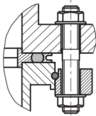
Abb. 11: Flanschverbindung ISO-K mit ISO-F, Stiftschraube und Durchgangsbohrung
