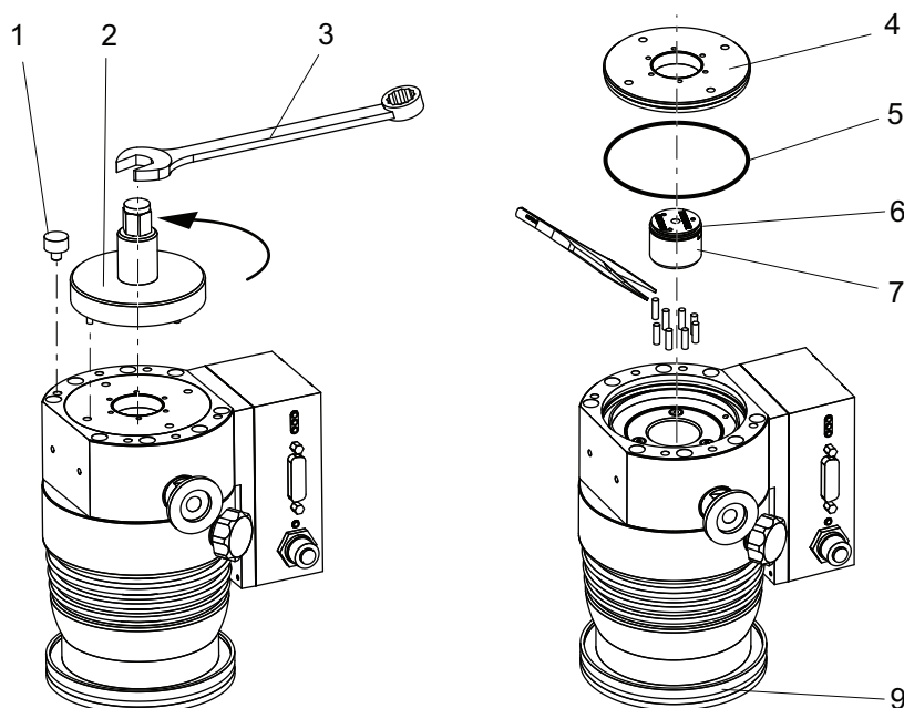
Abb. 19: Betriebsmittelspeicher demontieren
