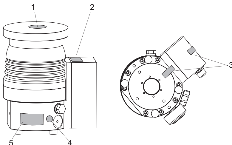
Abb. 2: Position der Aufkleber auf dem Produkt
