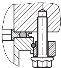
Abb. 9: Flanschverbindung ISO-K mit ISO-F, Sechskantschraube und Gewindebohrung
