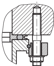
Abb. 10: Flanschverbindung ISO-K mit ISO-F, Stiftschraube und Gewindebohrung
