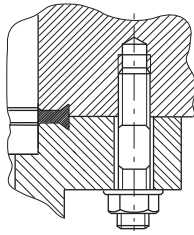
Abb. 13: Flanschverbindung CF-F, Stiftschraube und Gewindebohrung
