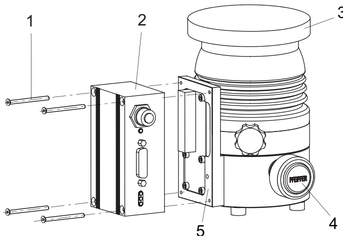
Abb. 21: Demontage und Montage der Antriebselektronik
