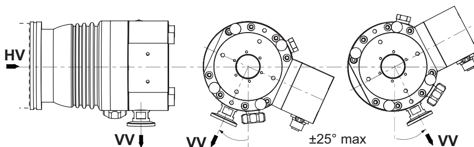
Abb. 5: Empfohlene Ausrichtung bei Verwendung ölgedichteter Vorpumpen
