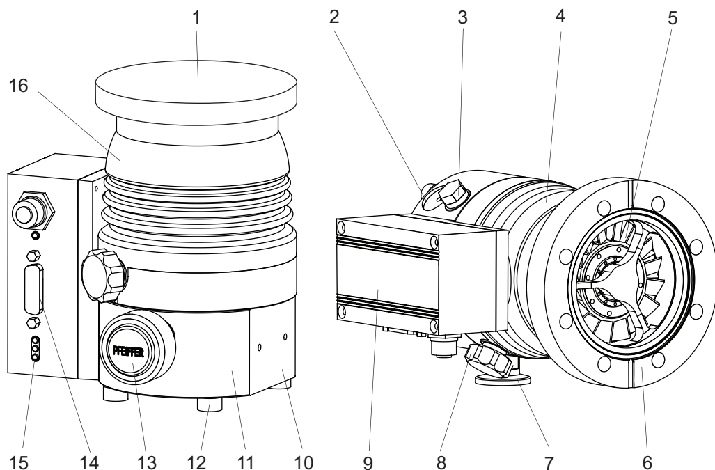
Abb. 3: Aufbau HiPace 80
