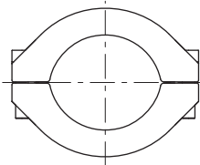
Abb. 6: Flanschverbindung ISO-KF mit Spannring
