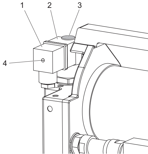
그림 7: 전기 연결 설정
