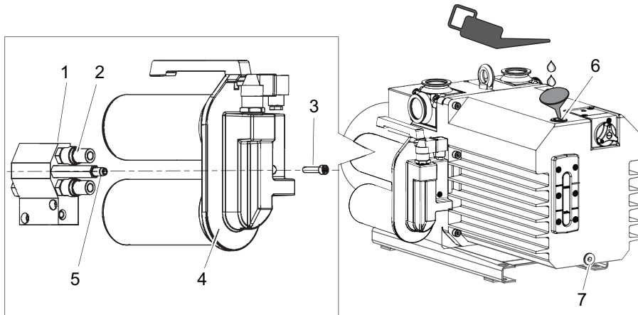
그림 6: 필터 캐리어 설치
