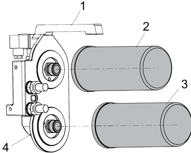
그림 13: 필터 카트리지 교체
