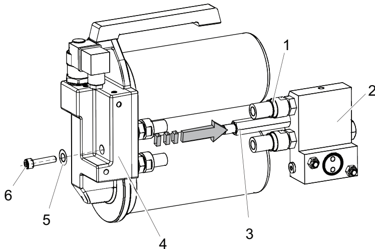
그림 3: 오일 필터 제거
