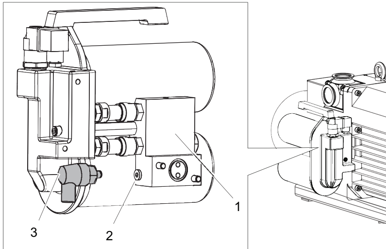
그림 9: 압력 스위치 나사
