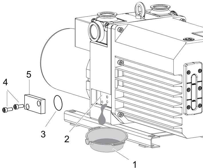
그림 4: 오일 덕트 커버 제거
