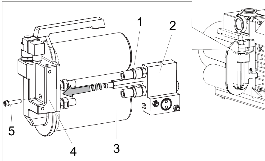
그림 12: 필터 캐리어 제거
