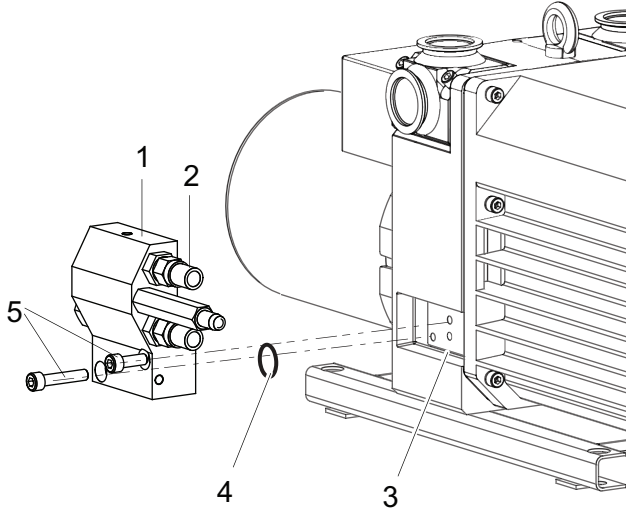
그림 5: 어댑터 장착
