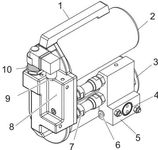
그림 2: 오일 필터의 구조
