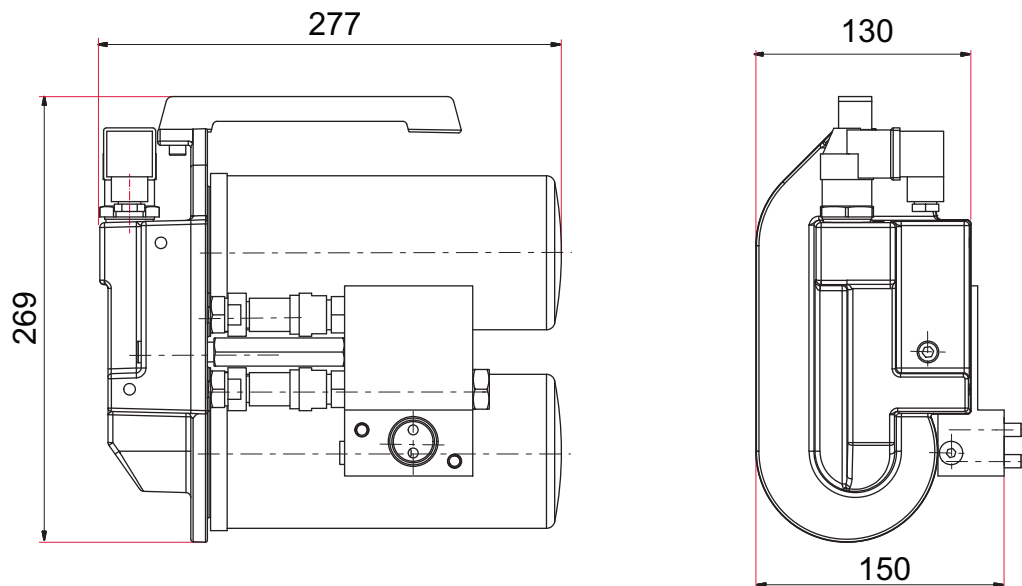
그림 14: 치수 OFC 35/65 치수(mm)
