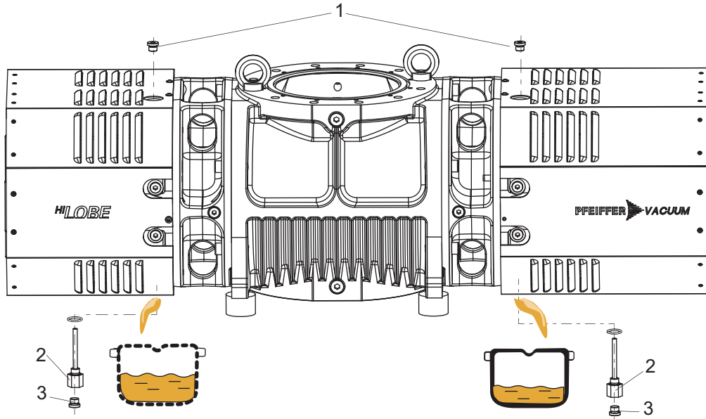
그림 16: 윤활유 배출하기
