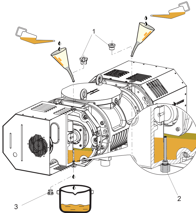
그림 8: 윤활유 충전
