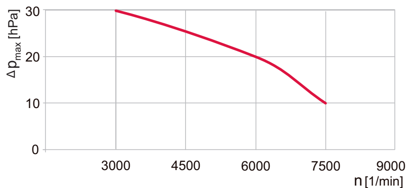
그림 2: 펌프 회전 속도에 따라, 입력 및 출력 영역 사이의 최대 허용 차압
