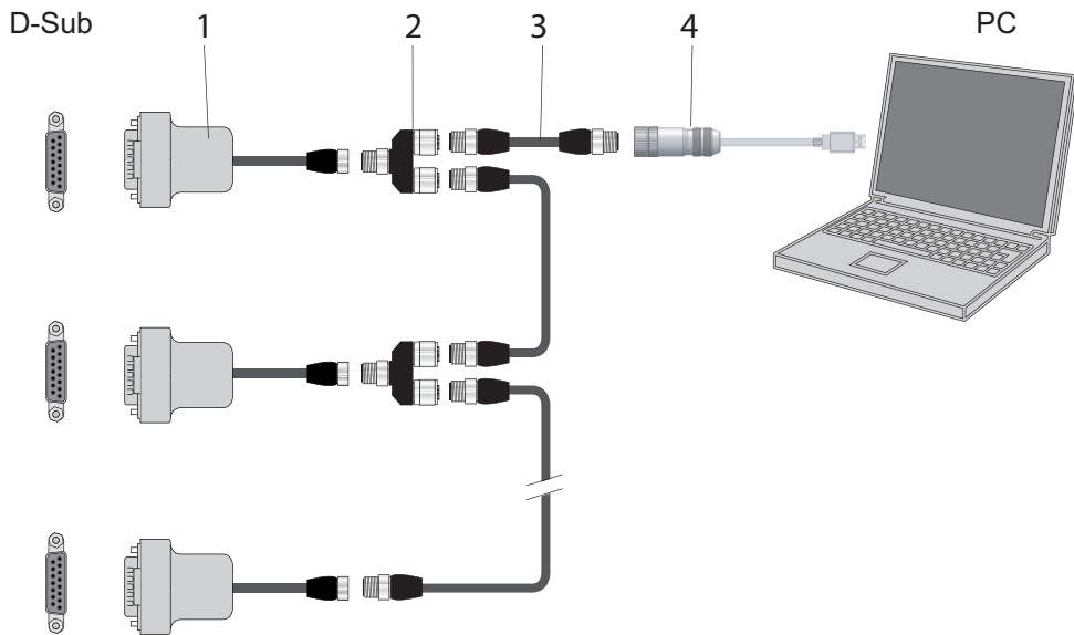
그림 14: 연결 케이블 및 액세서리를 사용하여 연결 RS-485를 통해 교차 결합
