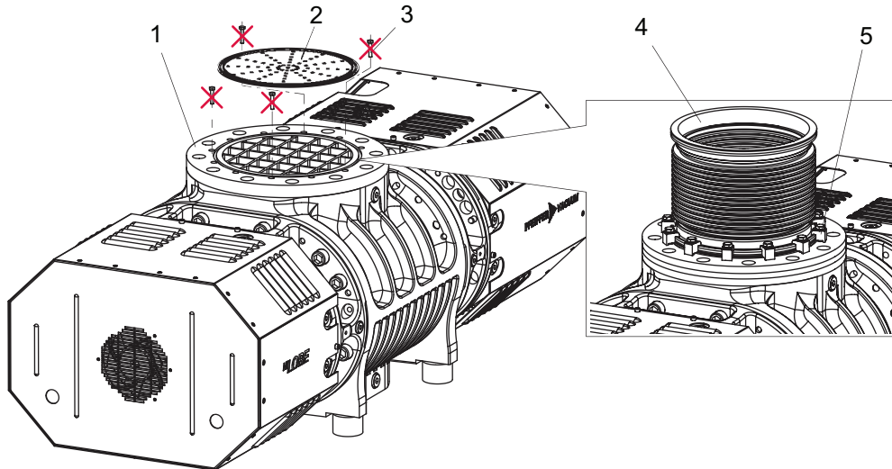
그림 9: 진공 영역을 ISO-F에 연결하기
