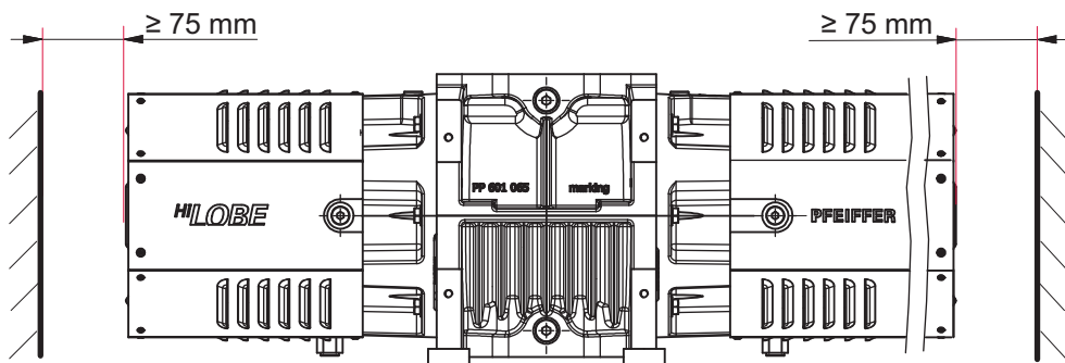
Abb. 7: Mindestabstände
