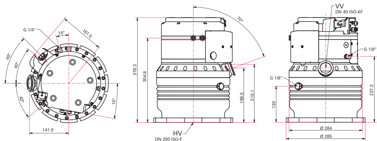
Fig. 34: HiPace 1200 U | DN 200 ISO-F
