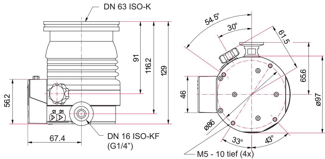
그림 21: HiPace 80 Neo | DN 63 ISO-K 치수(mm)
