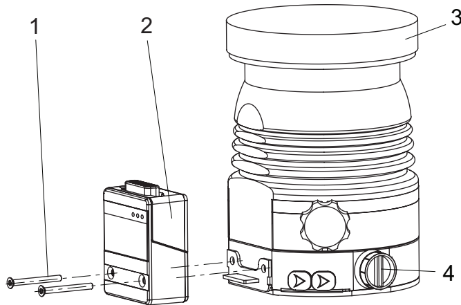
그림 18: 전자 드라이브 유닛 설치 및 제거
