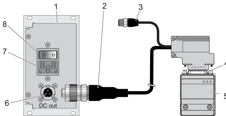
그림 15: 전자 드라이브 유닛을 전원 공급장치 팩에 연결하기
