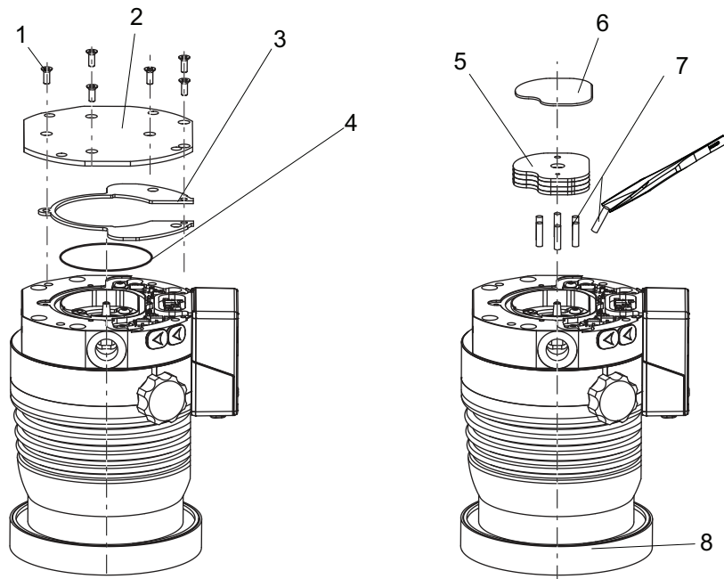
그림 16: 작동유 저장조 제거하기
