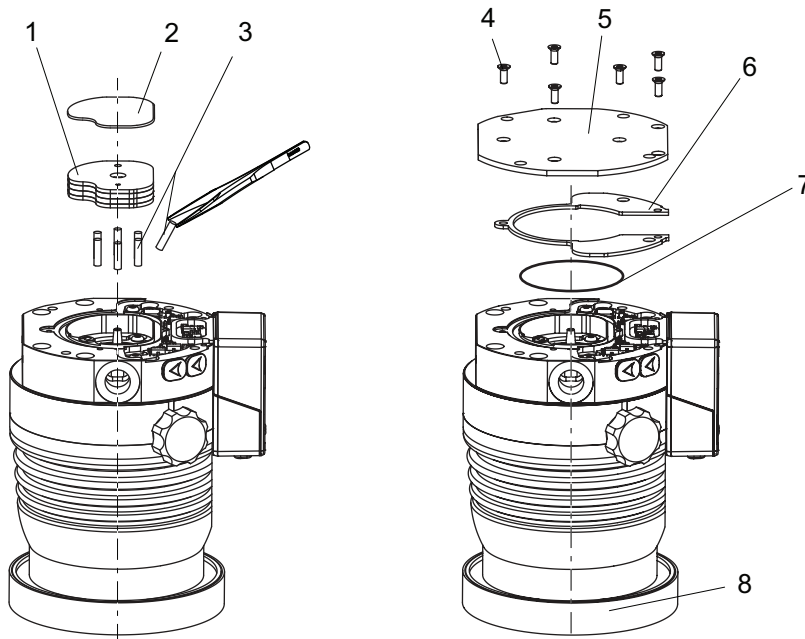
그림 17: 작동유 저장조 조립하기
