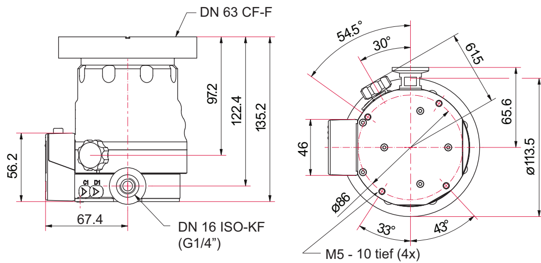
그림 22: HiPace 80 Neo | DN 63 CF-F 치수(mm)
