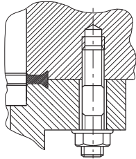
그림 8: 플랜지 연결 CF-F, 스테드 나사 및 탭 구멍
