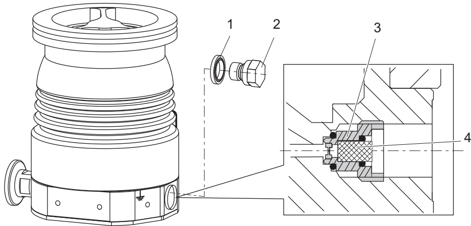
그림 13: 내부 밀봉 가스 스로틀(옵션)
