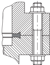
그림 9: 플랜지 연결 CF-F, 스테드 나사 및 관통 구멍
