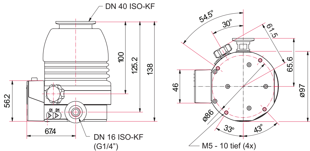
그림 20: HiPace 80 Neo | DN 40 ISO-KF 치수(mm)
