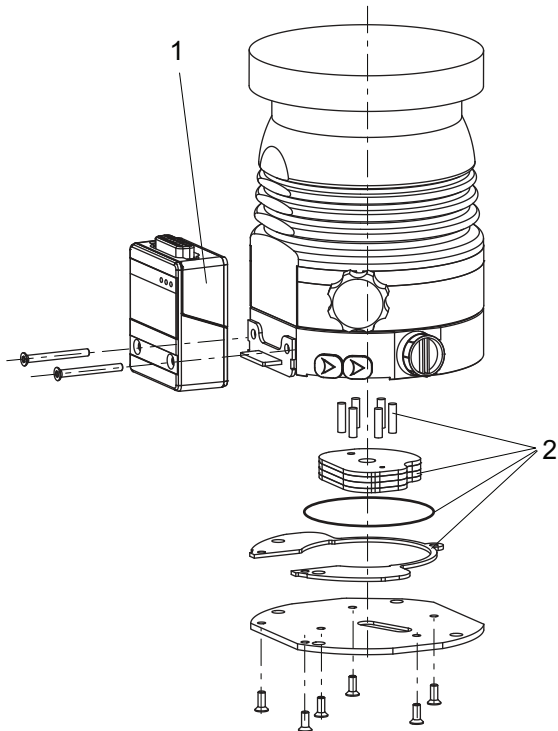
그림 19: 예비 부품, HiPace 80 Neo
