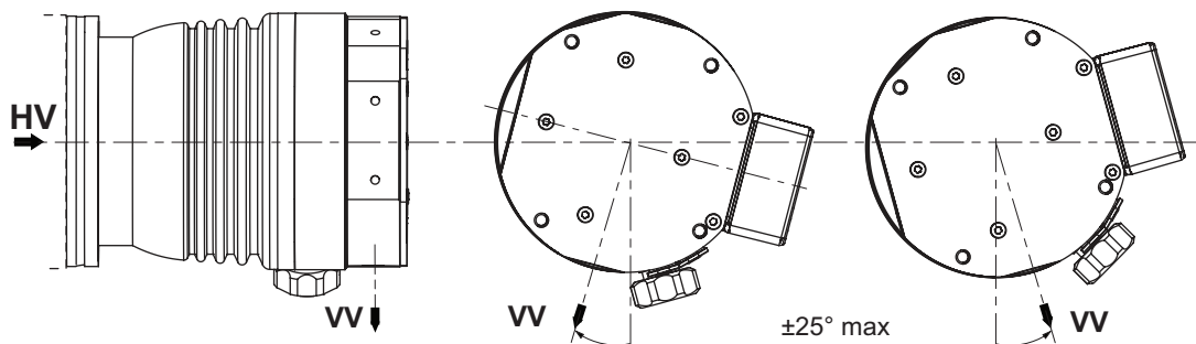
그림 4: 오일 밀봉 배압 펌프 사용 시 권장되는 정렬
