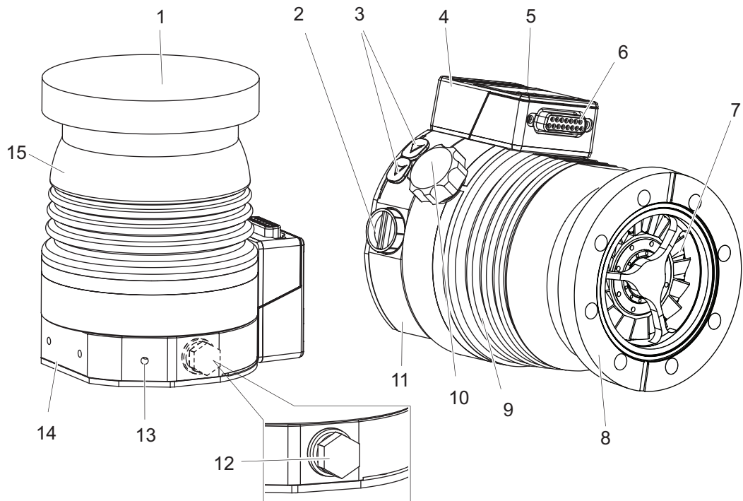
그림 2: HiPace 80 Neo 설계
