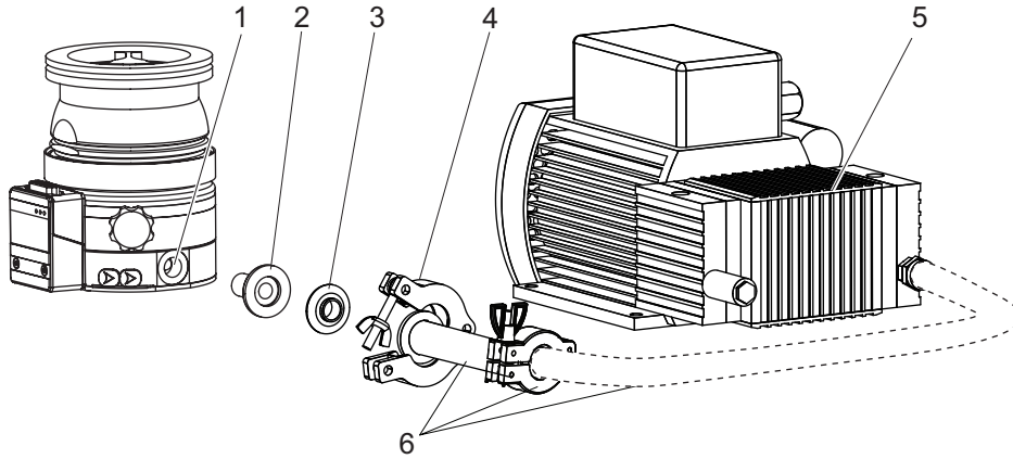
그림 10: MVP에서 전진공 연결의 예
