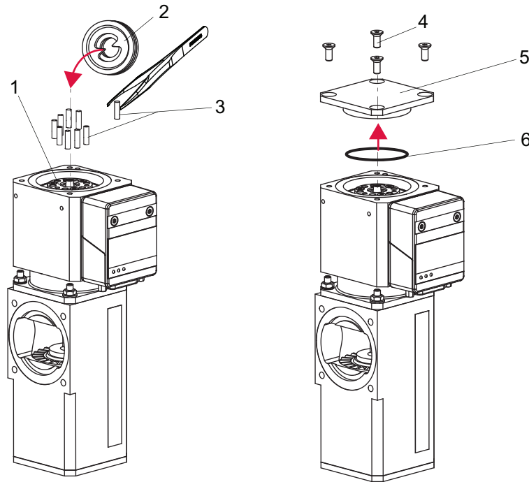
그림 13: 작동유 저장조 조립하기
