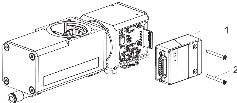
그림 14: 전자 드라이브 유닛 TC 80 설치 및 제거
