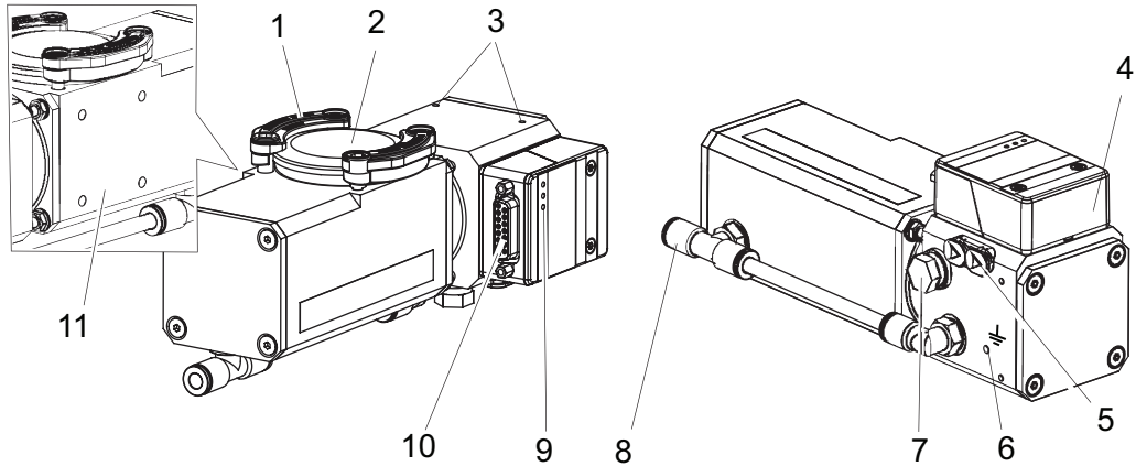
그림 2: HiPace 10 Neo 설계
