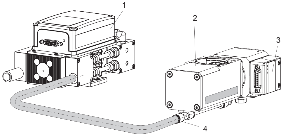
그림 6: HiPace 10 Neo의 전진공 연결부의 예
