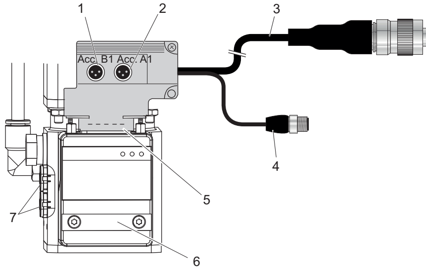
그림 7: 연결 케이블을 통한 액세서리 연결부
