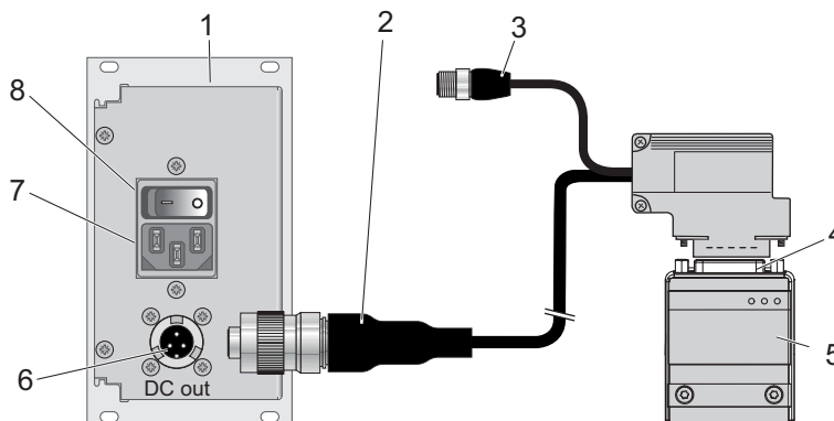
그림 9: 전자 드라이브 유닛을 전원 공급장치 팩에 연결하기
