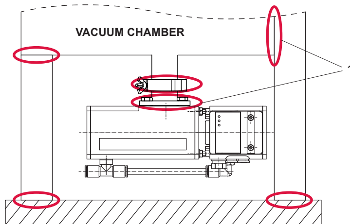
그림 3: 예시: 외부 진동으로 인한 변위 및 기울어짐 방지하기
