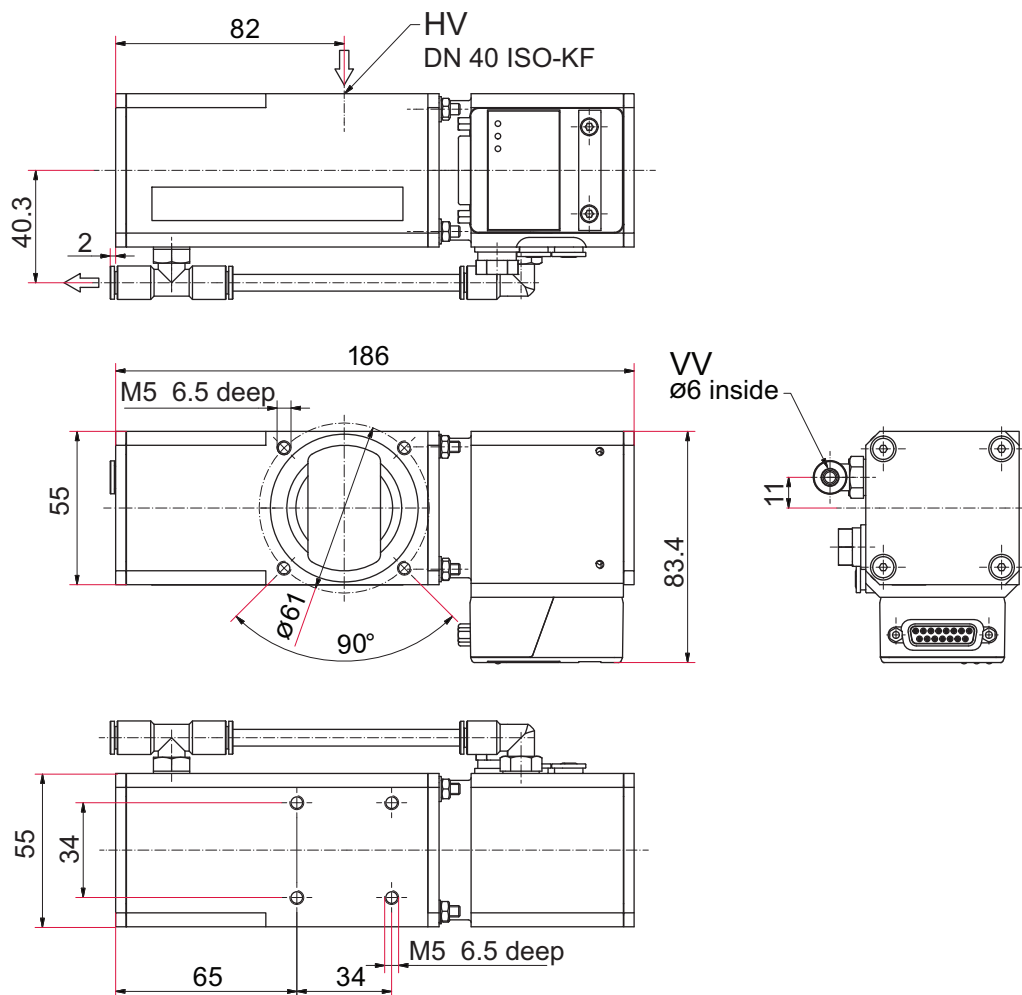
그림 16: HiPace 10 Neo | TC 80 | DN 40 ISO-K 치수(mm)
