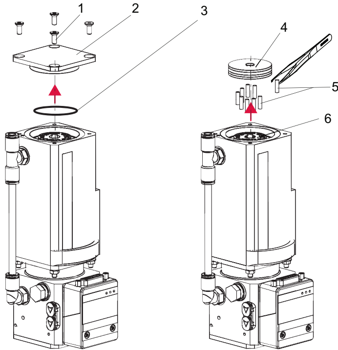
그림 10: 작동유 저장조 제거하기
