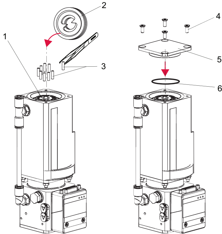
그림 11: 작동유 저장조 조립하기
