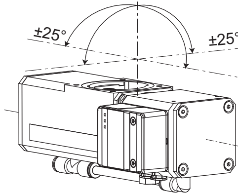
그림 4: 오일 밀봉 배압 펌프 사용 시 권장되는 전진공 연결부 정렬
