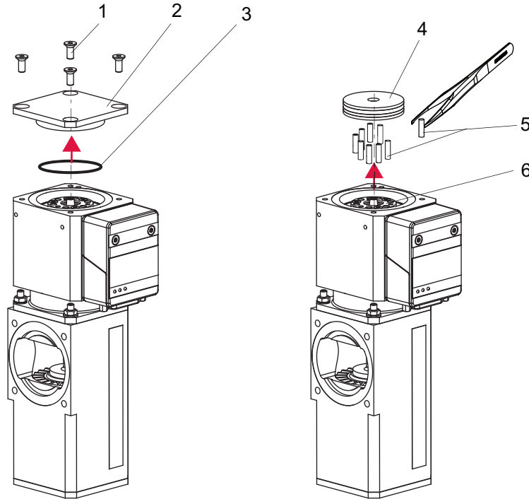
그림 12: 작동유 저장조 제거하기
