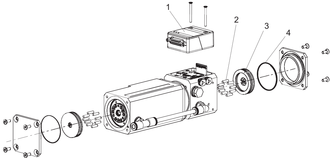
그림 15: 예비 부품, HiPace 10 Neo
