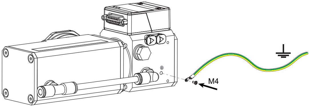
그림 8: 예시: 접지 케이블 연결
